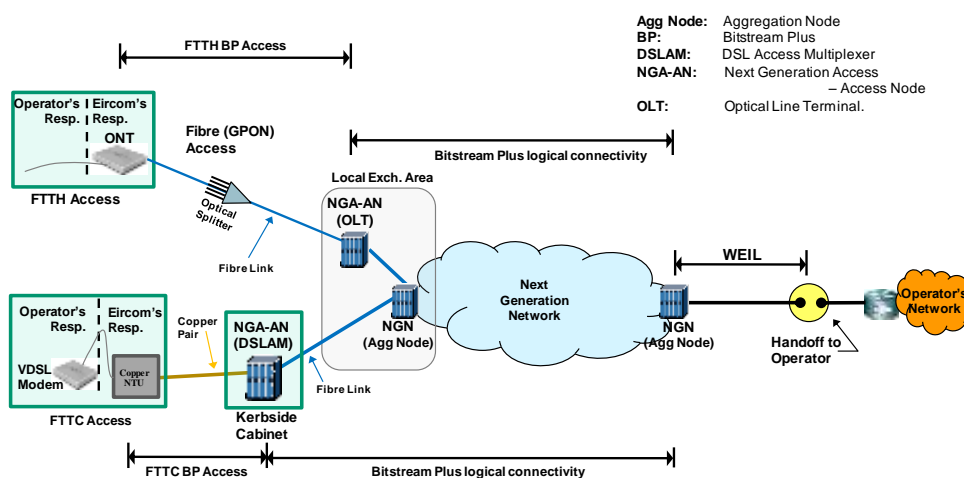
Figure 2: open eir NGA Bitstream Plus
